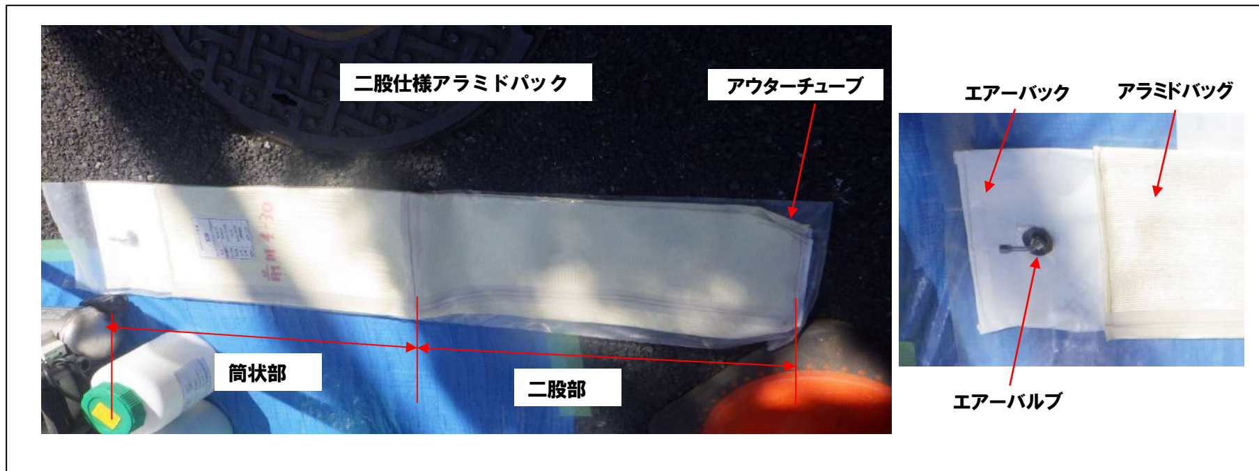
【 二又仕様の膨張前 】
